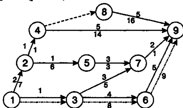
Рис. 24.1. Сетевой график
